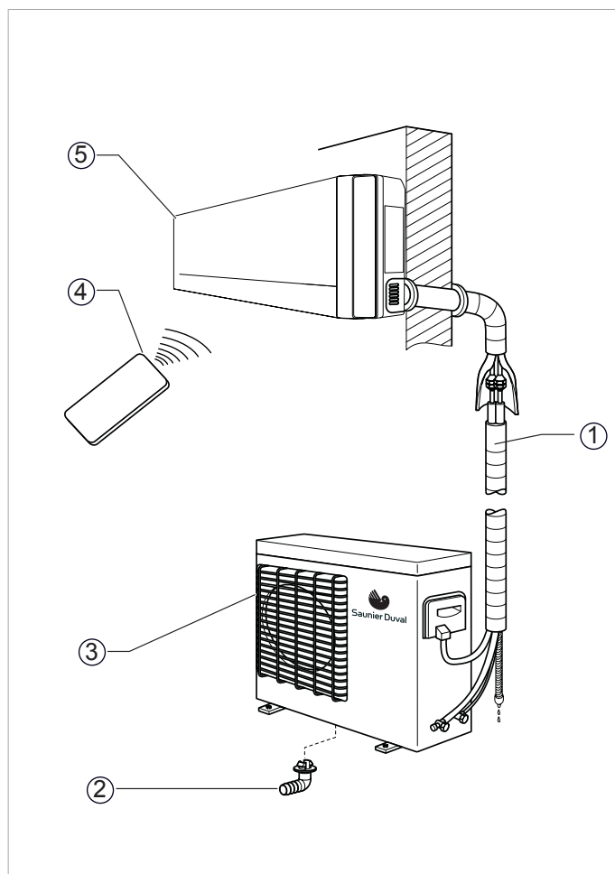
Rys. 5.1 Podzespoły klimatyzatora.
