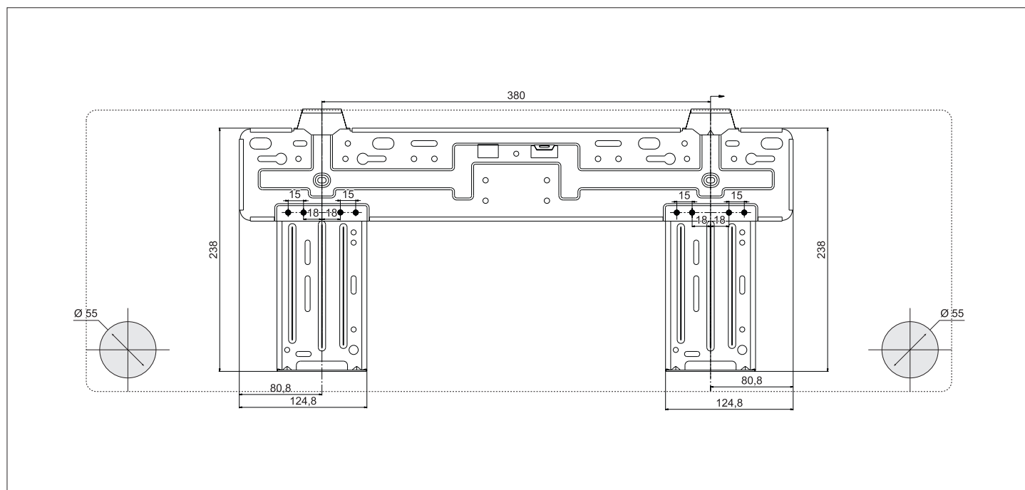
Fig. 9.7 Płyta montażowa dla modelu 17-035 NMWI.
