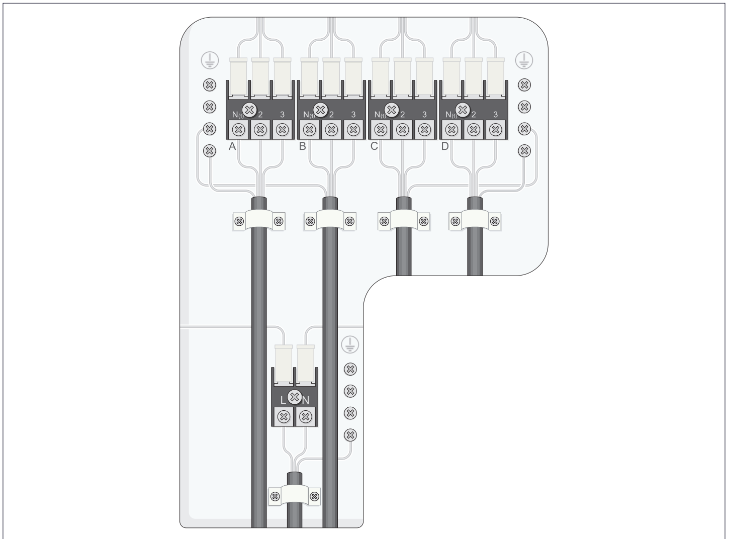
Fig. 11.2 Podłączenie zasilania elektrycznego jednostki zewnętrznej.
