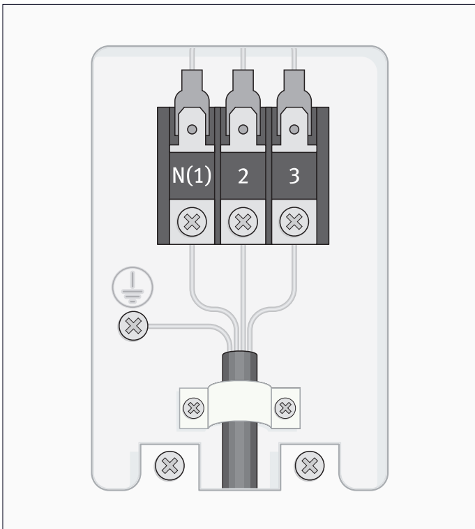
Fig. 11.2 Podłączenie zasilania elektrycznego jednostki zewnętrznej.
