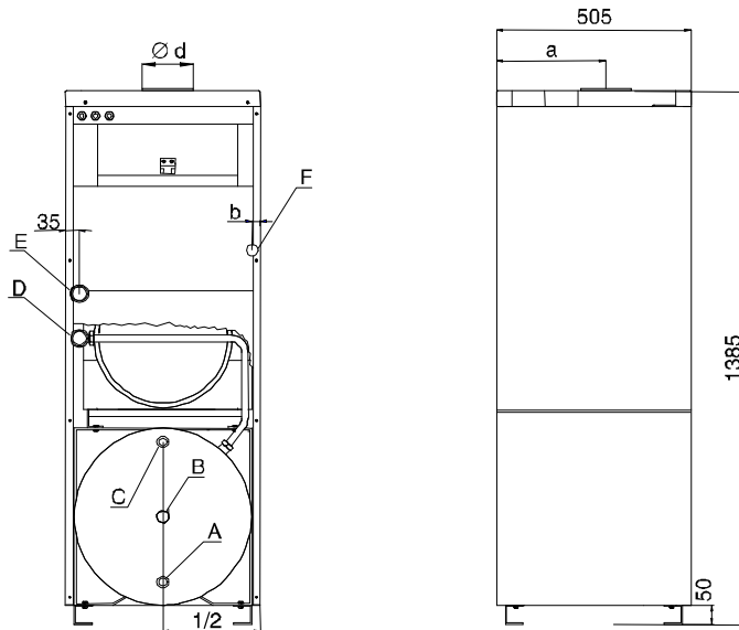
Rys. 1 Wymiary podstawowe i przyłączeniowe
