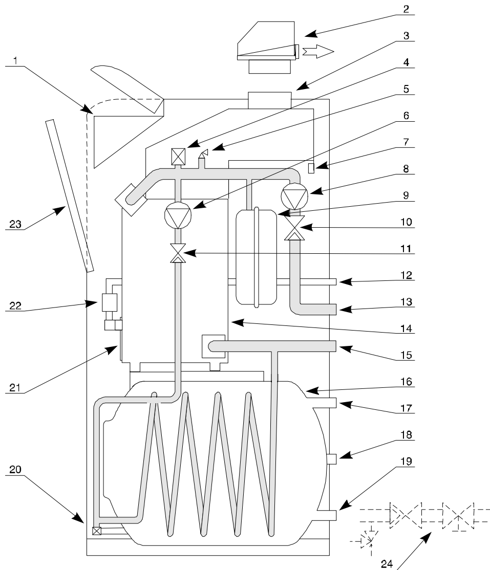
Rys. 2 Schemat roboczy kotła
